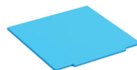
sky: color code SB
